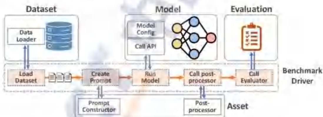
图 9 大模型基准测试工具 LLMeBench 框架图
